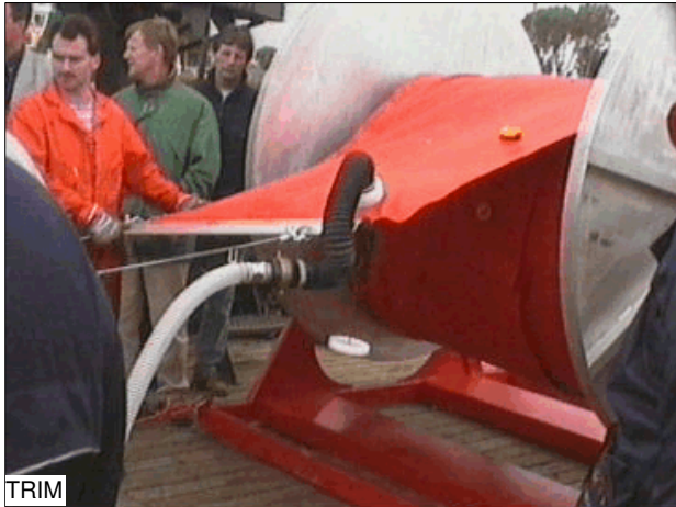
"Oil Stop" scherm op haspel
