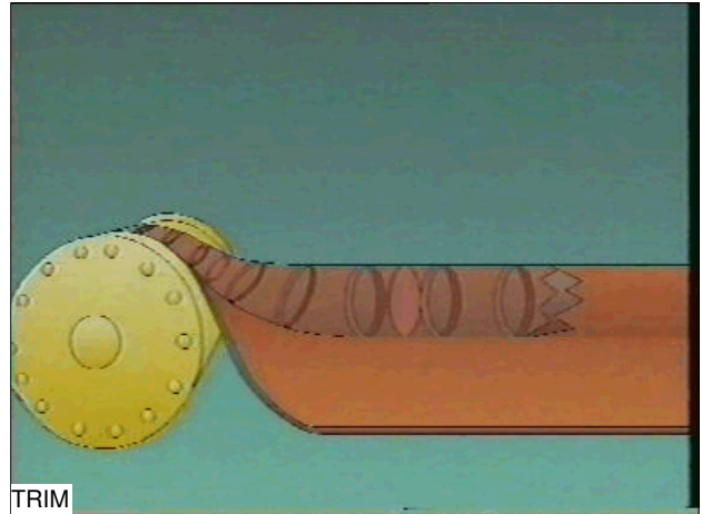
Principe zelfluchtaanzuigend systeem
