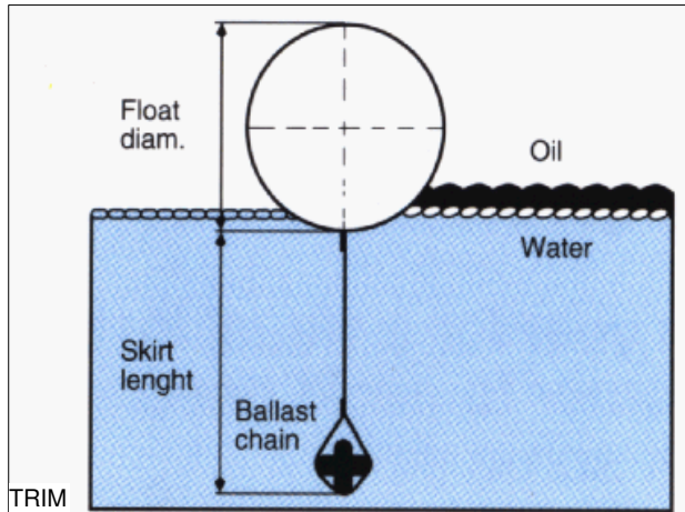
Dwarsdoorsnede Collapsible
